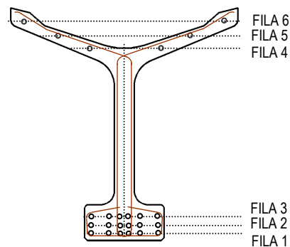
Sección Armadura
