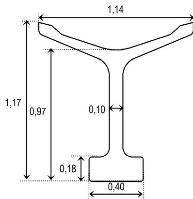
Sección Transversal
